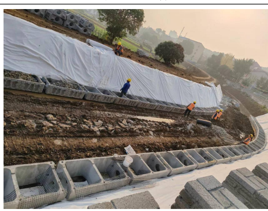
阶梯式生态挡墙
