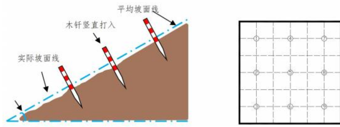
图 4-1 测钎法示意图
